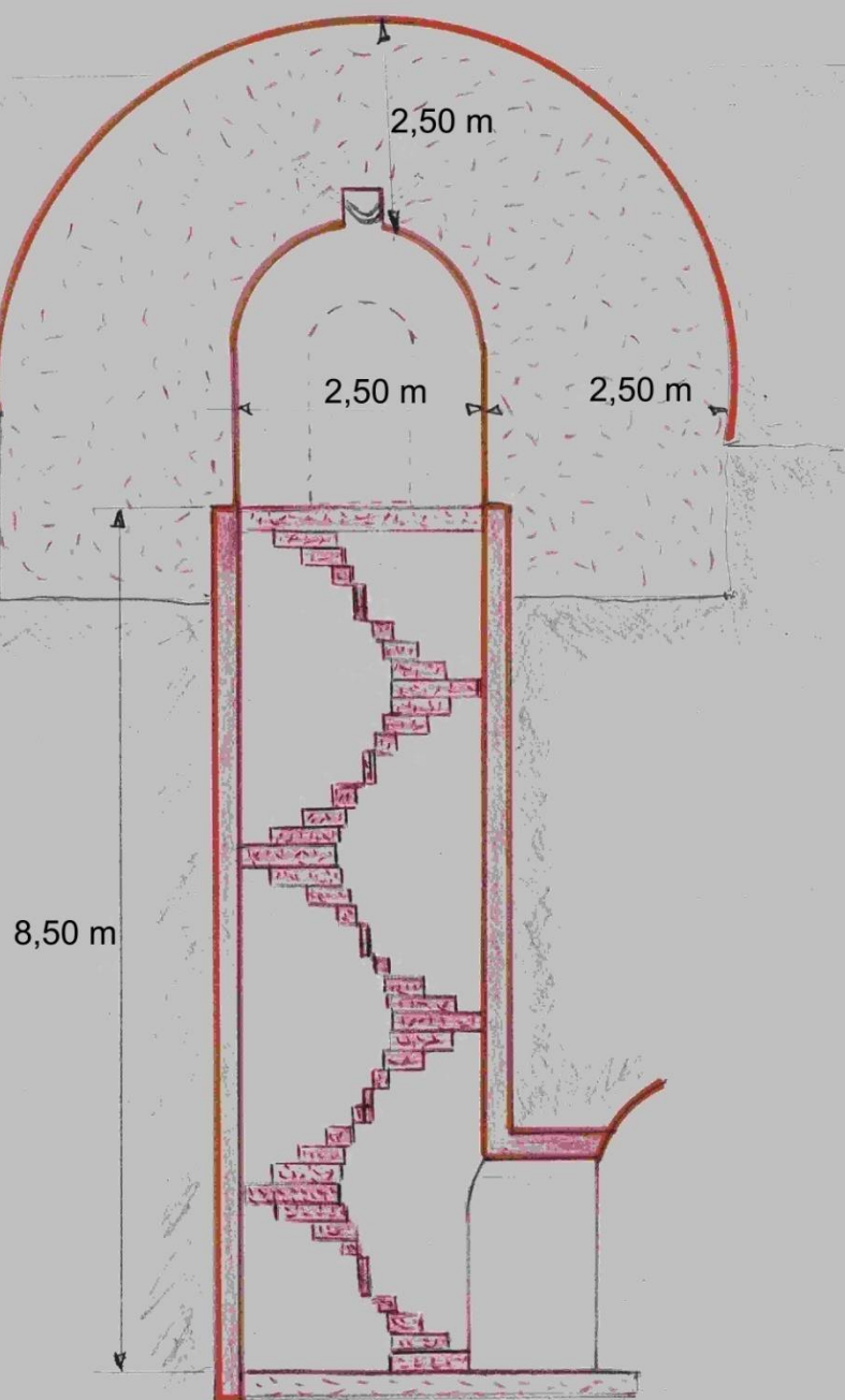
Puit d'escalier à vis
