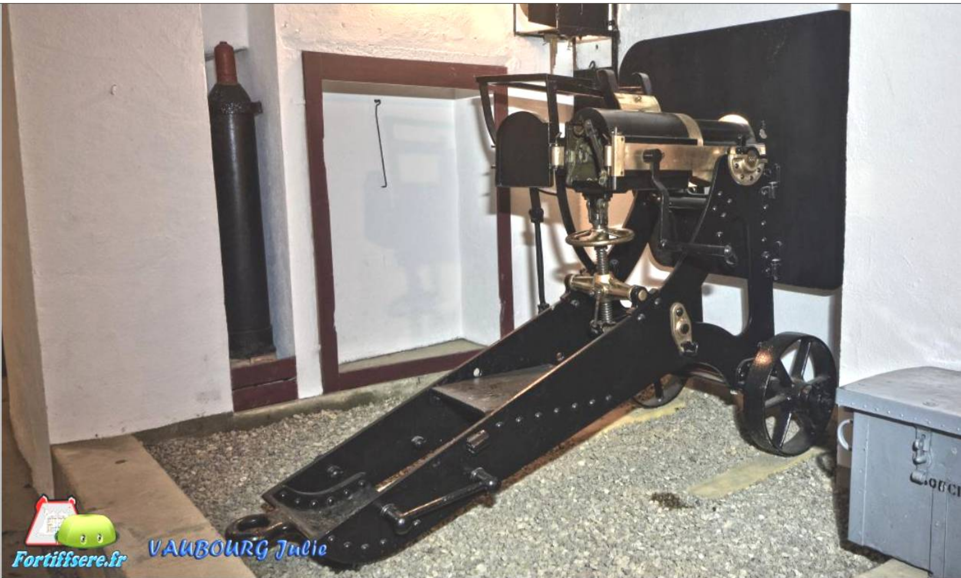
Le canon revolver dans le coffre simple du fort de Villey le Sec à Toul. Cliché VAUBOURG Julie
