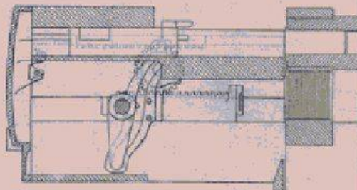
Chargement et extraction (7/3)
